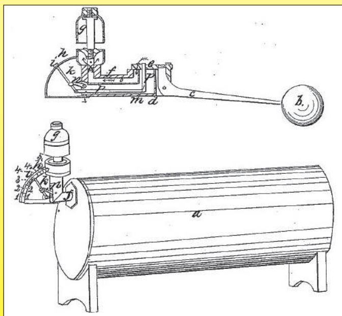
Joseph Dilks, brevet US7808, Décembre 1850, indicateur de niveau à flotteur avec sifflet d'alarme à vapeur
