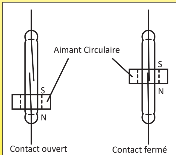
A1 : Modèle vertical
