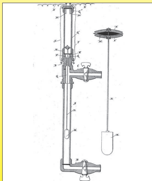
Mac Dermott, Détecteur de niveau à flotteur vertical avec contact haut et bas pour chaudière, Brevet US 487634, Décembre 1892
