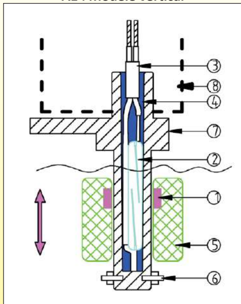
A1 : Modèle vertical
