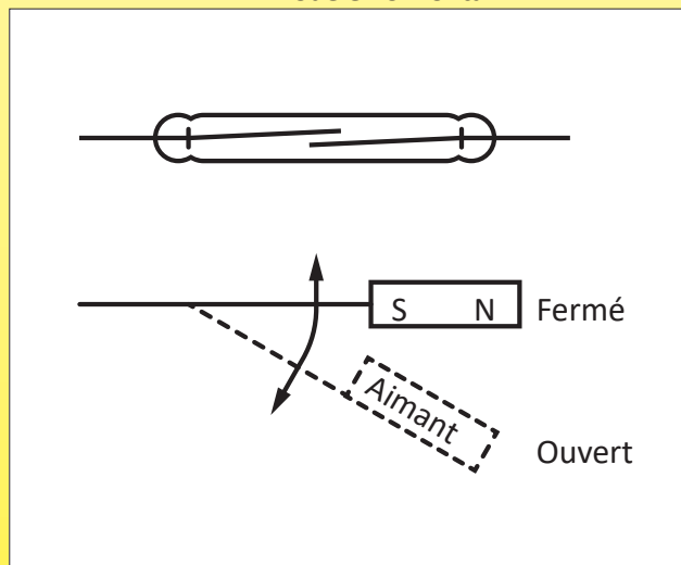
A2 : Modèle horizontal
