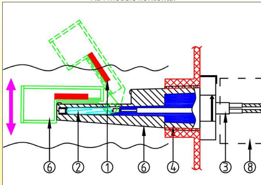
A2 : Modèle horizontal
